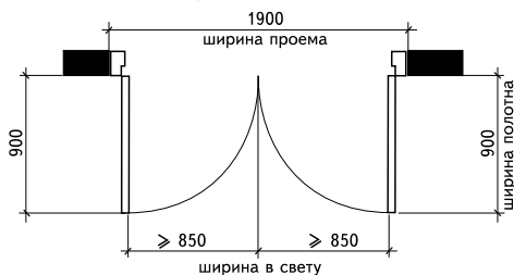
Рис. 6.7 Двустворчатая симметричная дверь НЕУДОБНО
