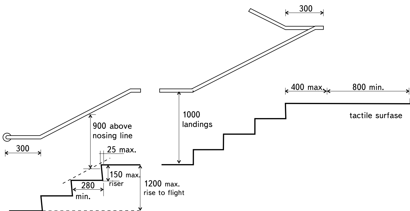
Рис. 8.40. Лестница наружная
